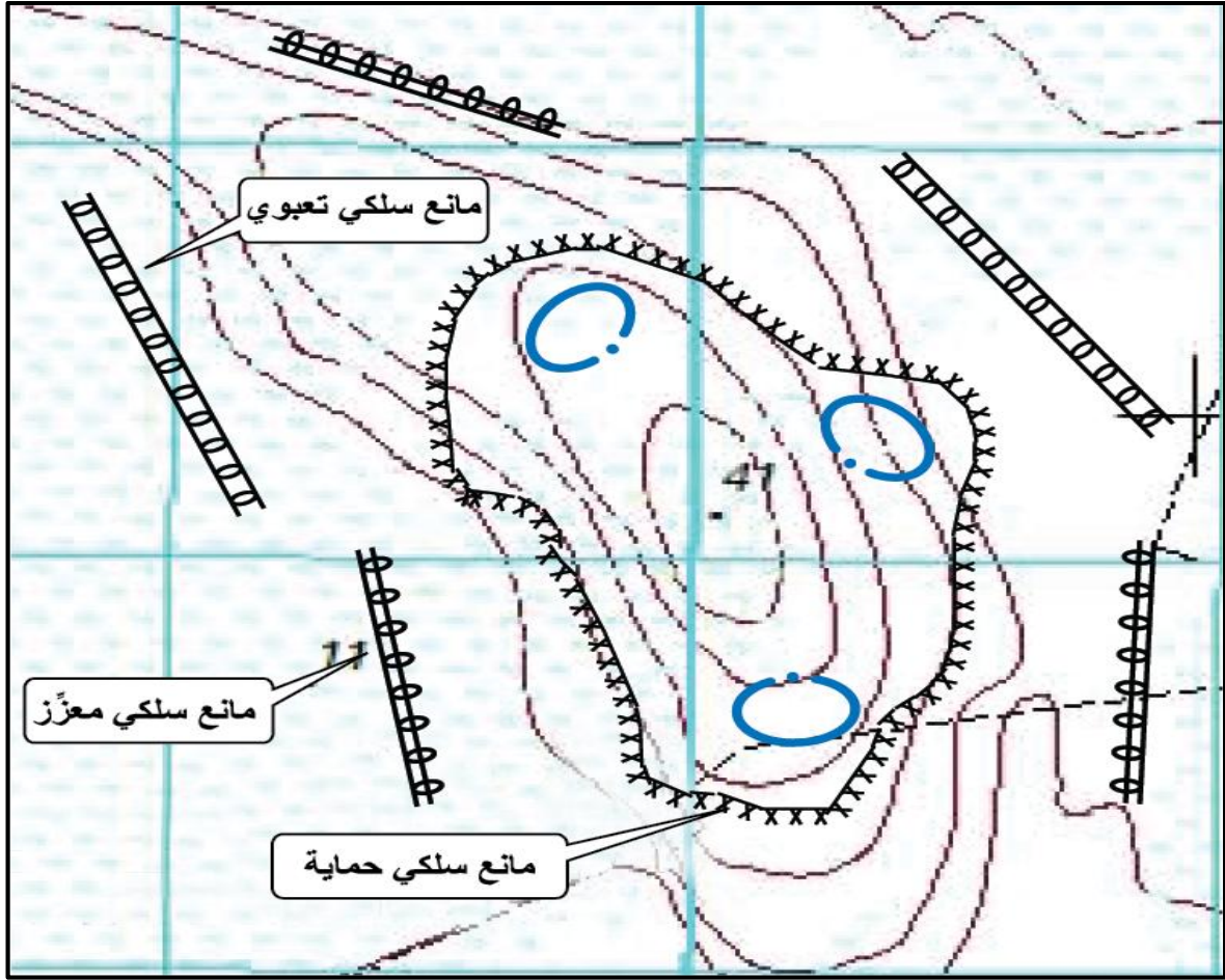
الشكل رقم (25) مثال على الأنواع الثلاثة من الموانع السلبيه
